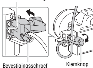
Bevestigingsschroef
